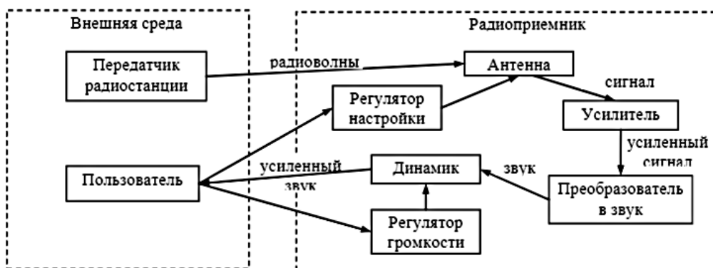
Рисунок 5.2 – Структура радиоприемника
