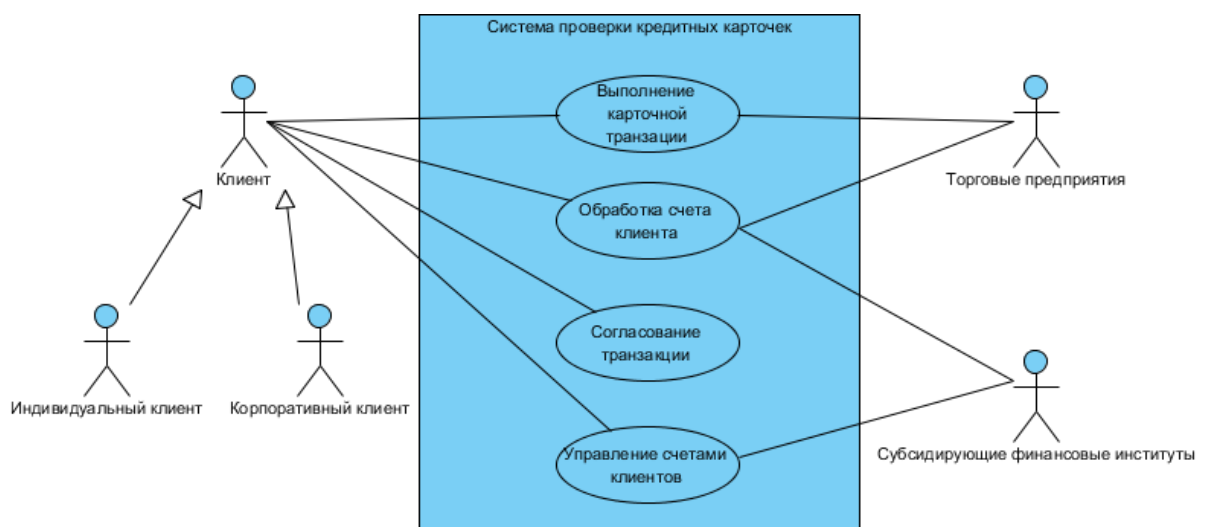
Рисунок 4.11 – Моделирование контекста системы
